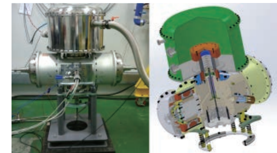
〈대용량 스터링 극저온 냉동기〉
